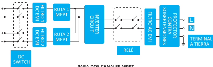
PARA DOS CANALES MPPT
