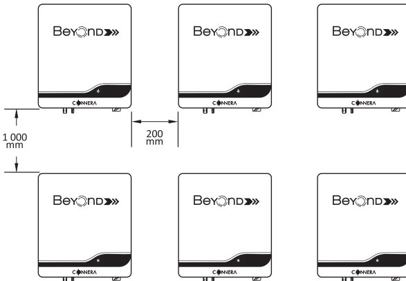
INSTALACIÓN DE MÚLTIPLES INVERSORES EN MODO APILADO
