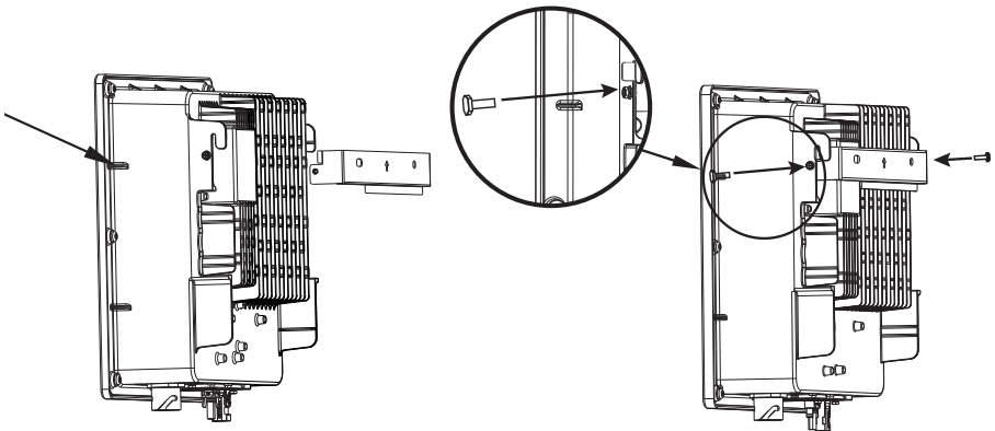
Montar el soporte para pared
