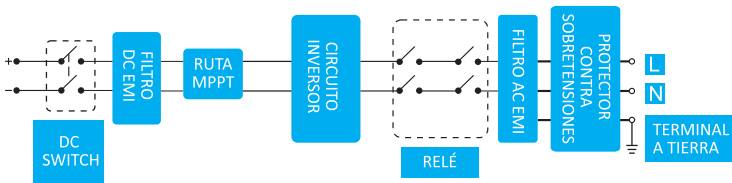
PARA UN CANAL MPPT
